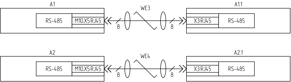
Цепи связи терминала с ИЧМ
